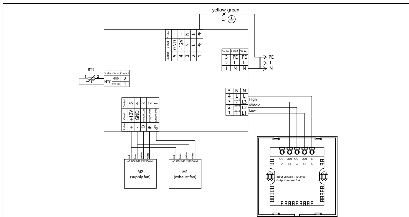
Fig. 12. Wiring diagram
